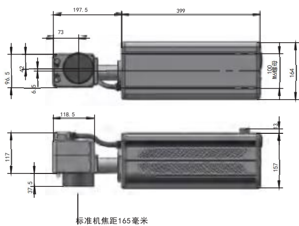
激光头尺寸:
