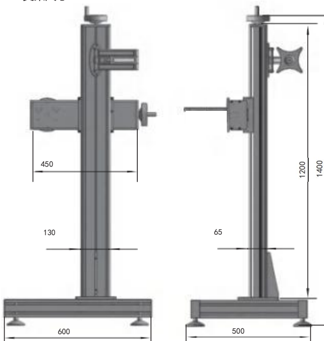
支架尺寸:
